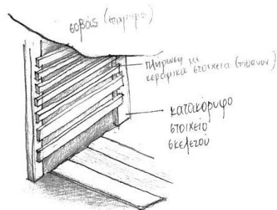
μπαγδατί, σκίτσο. κατασκευαστική μέθοδος εσωτερικών τοιχοποιιών.
