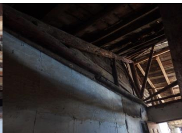
(2) Μπαμπάς, μπαμπατζάκι, αντηρίδες και γρεντιά, φωτογραφία στέγης.
