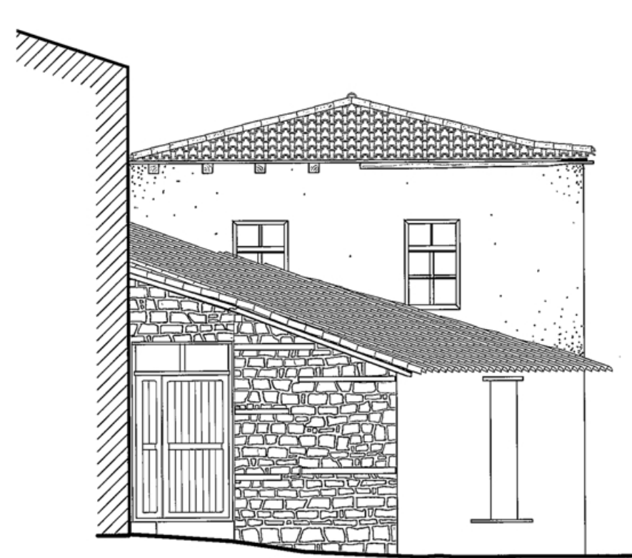
ΑΝΑΤΟΛΙΚΗ ΟΨΗ
