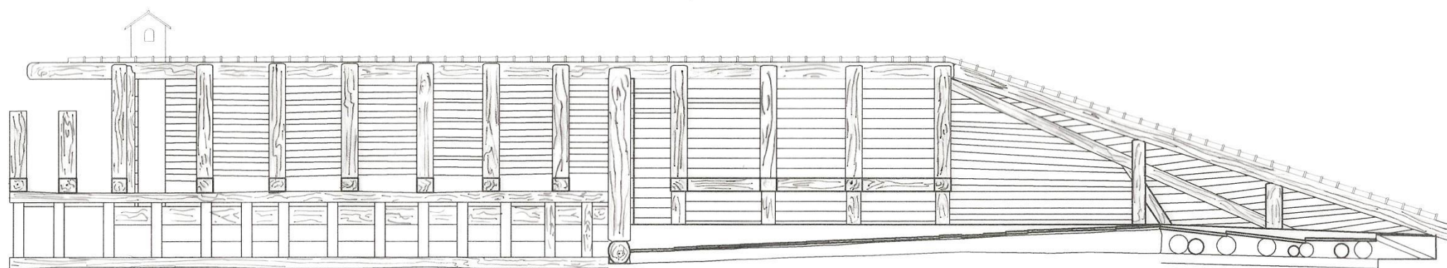
τομή στέγης
