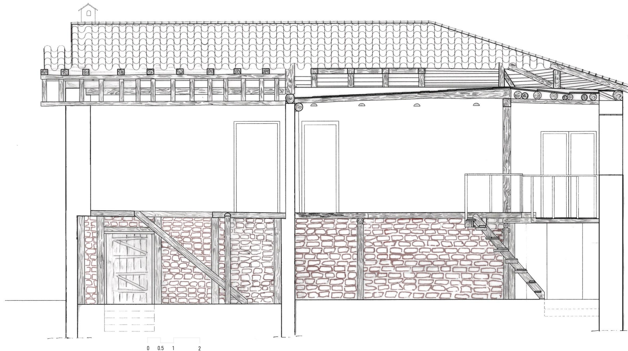
τομή 03
