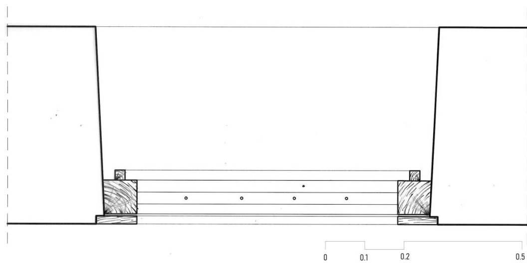
τομή Ε-Ε Π5
