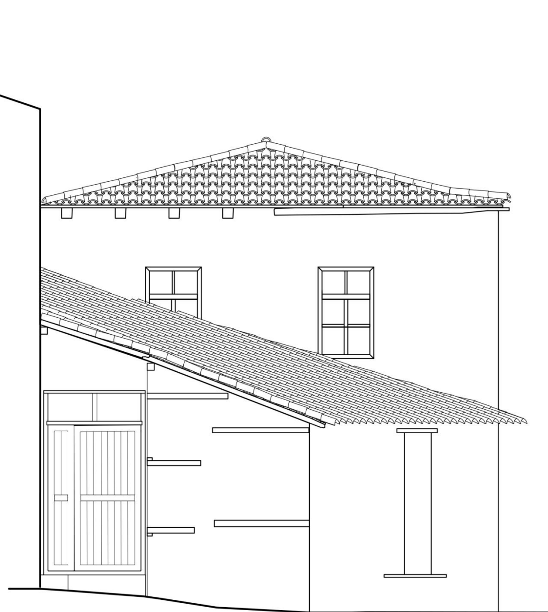
βορειοανατολική όψη
