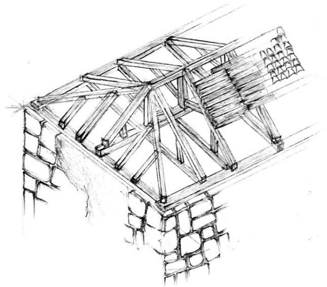
Προοπτικό σκίτσο στέγης.
