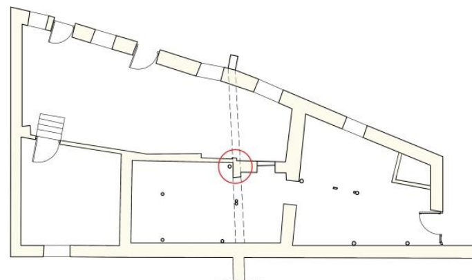
κάτοψη ισογείου
