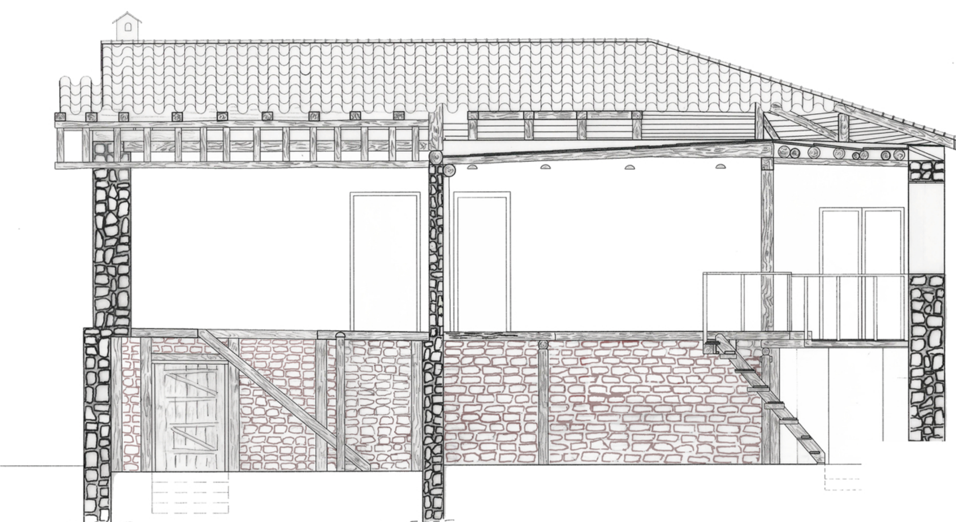
ΤΟΜΗ Β-Β'
