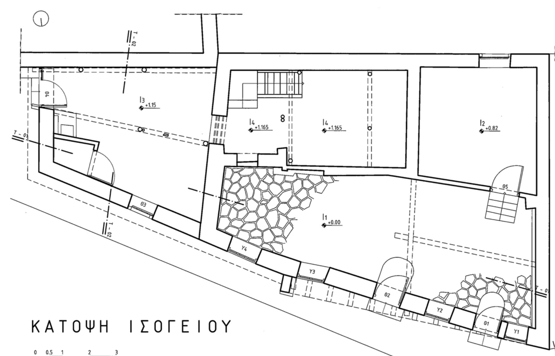
ΚΑΤΟΨΗ ΟΡΟΦΟΥ
