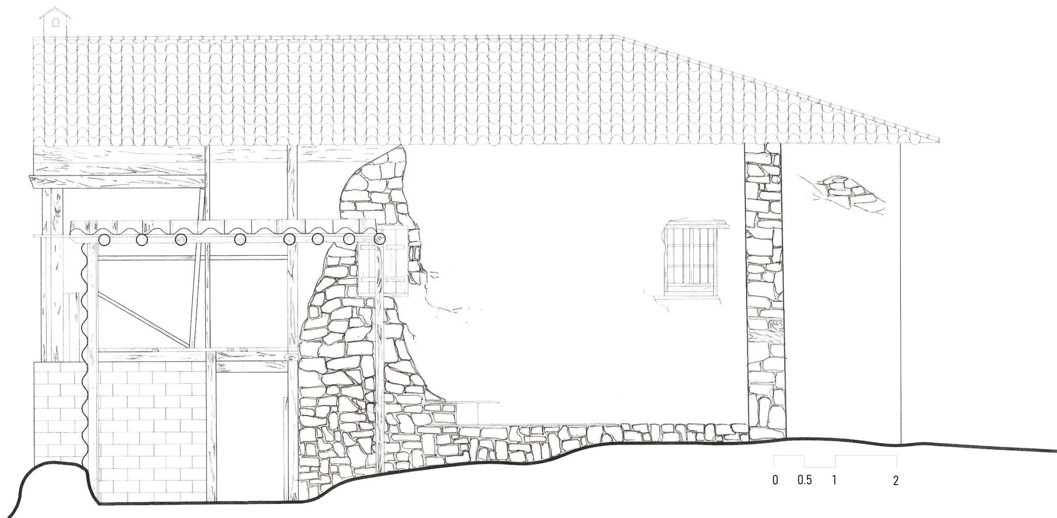
νότια όψη
