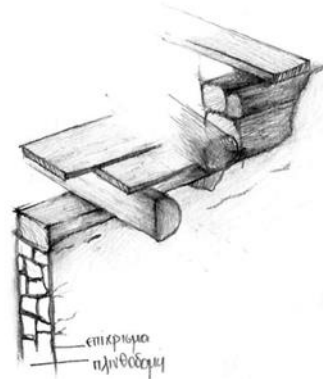
ανάλυση τοίχου στον όροφο, σκίτσο. νταμπάνια (δοκοί παράλληλες με τον τοίχο), γκρεντιές (δοκοί κάθετες στον τοίχο).
