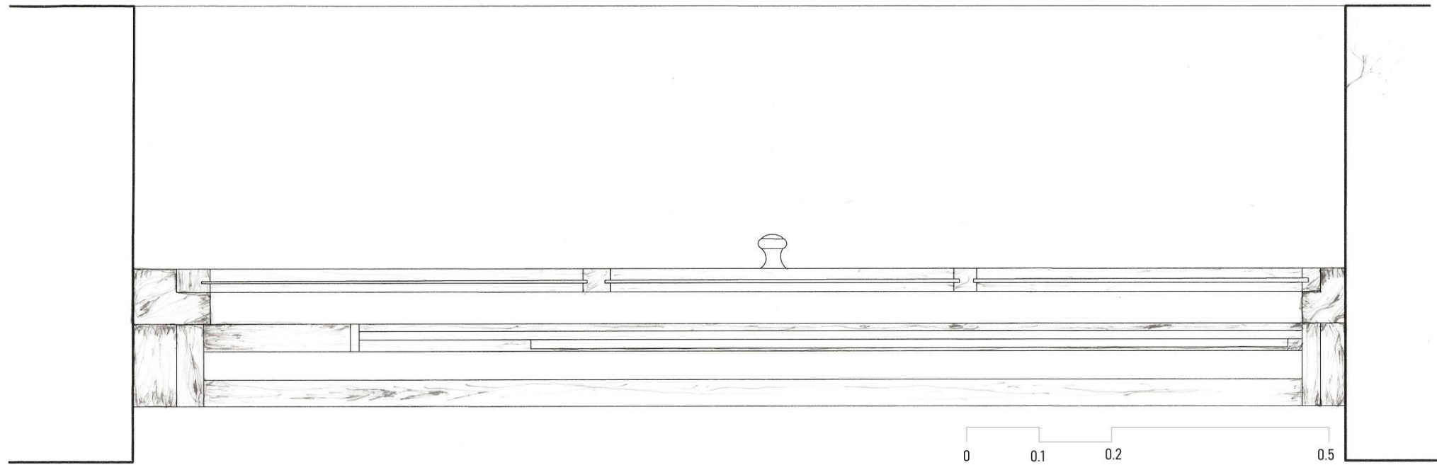
διαμήκης τομή Π3
