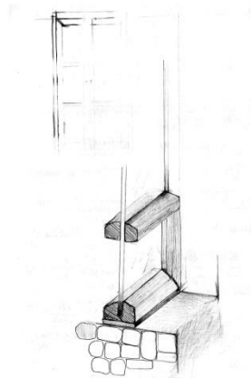
ανάλυση ανοιγόμενου δίφυλλου παραθύρου, σκίτσο. καρφωτό με ενσωματωμένο υαλοστάσιο.
