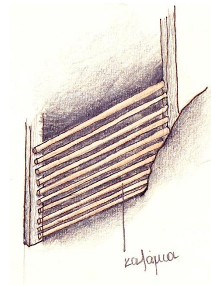
Λεπτομέρεια μπαγδατιού, σκίτσο
