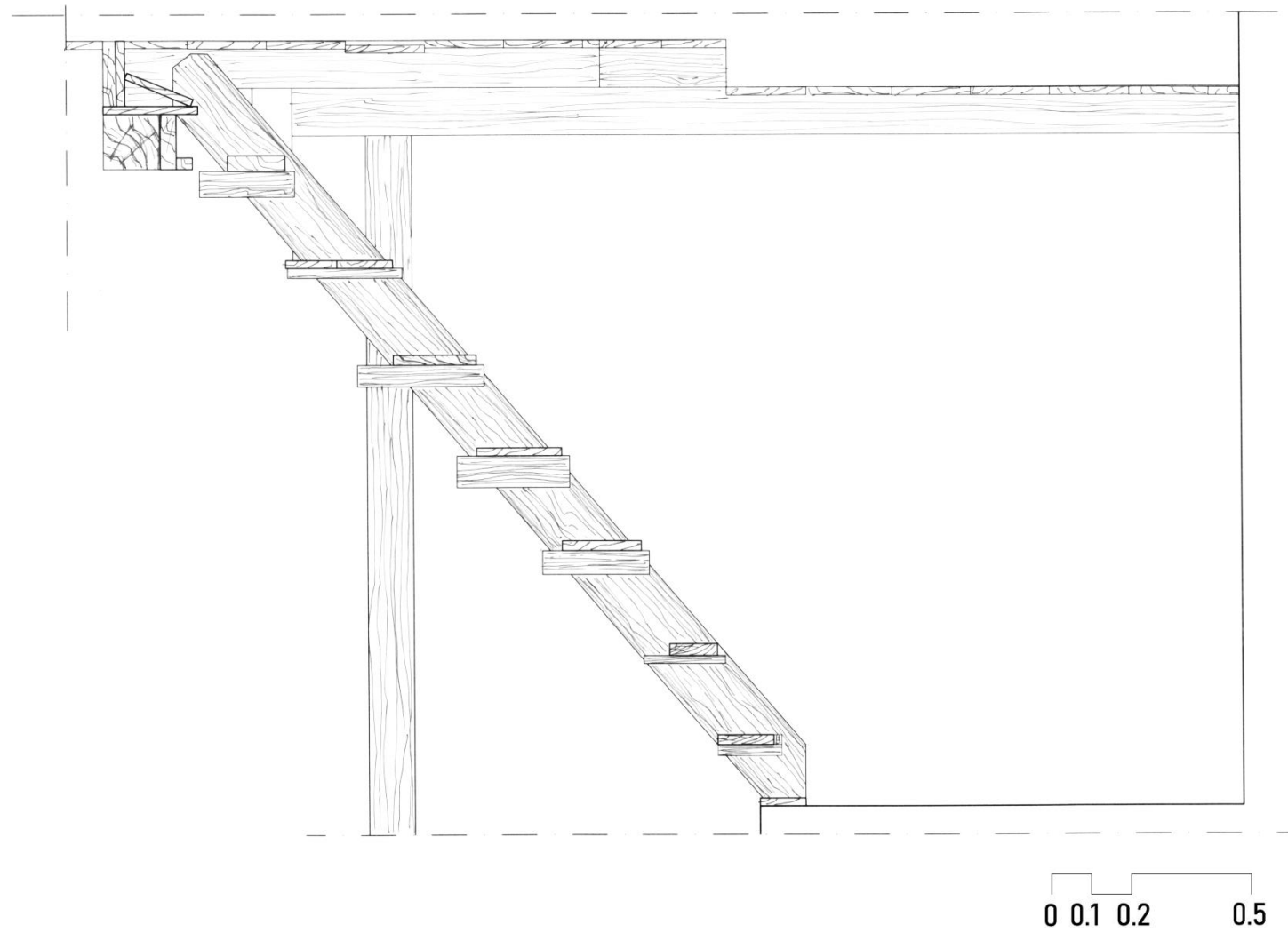
τομή σκάλας
