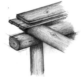
ανάλυση δαπέδου ορόφου, σκίτσο. ντιρέκι (στύλος) που στηρίζει το νταμπάνι (οριζόντια δοκός), πάνω στο οποίο «κάθεται» η γρεντιά (δοκός κάθετη στο νταμπάνι) και απλώνονται δύο σειρές από σανίδες.
